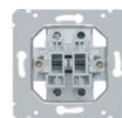
fitting, arrangement 11 double switching controller 10 AX, 250 V AC Ize použit jako žaluziový ovladač bez blokace
