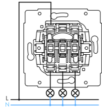
switch arrangement 1+1+1
