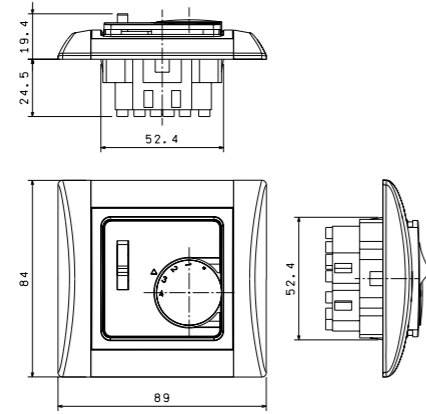
analog thermostat OREG/EBERLE DSE 2T/3T
